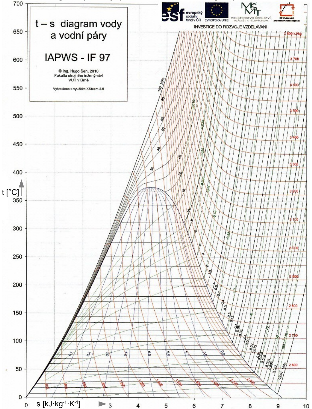
797 t-s diagram vody a vodní páry
