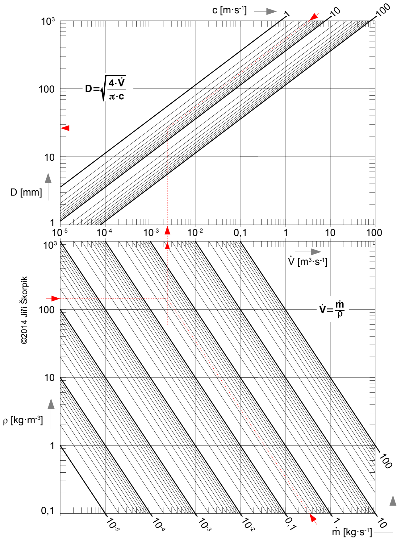
1039 Nomogram pro výpočet průměru potrubí
