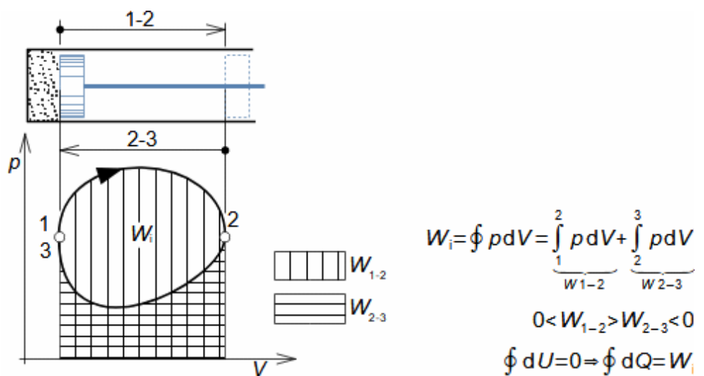
11: p - V diagram tepelného oběhu realizovaný v pístovém stroji W_{1-2} [J] práce vykonaná plynem během pohybu pístu z polohy 1 do polohy 2; W_{2-3} [J] práce vykonaná plynem během pohybu pístu z polohy 2 do polohy 3.
