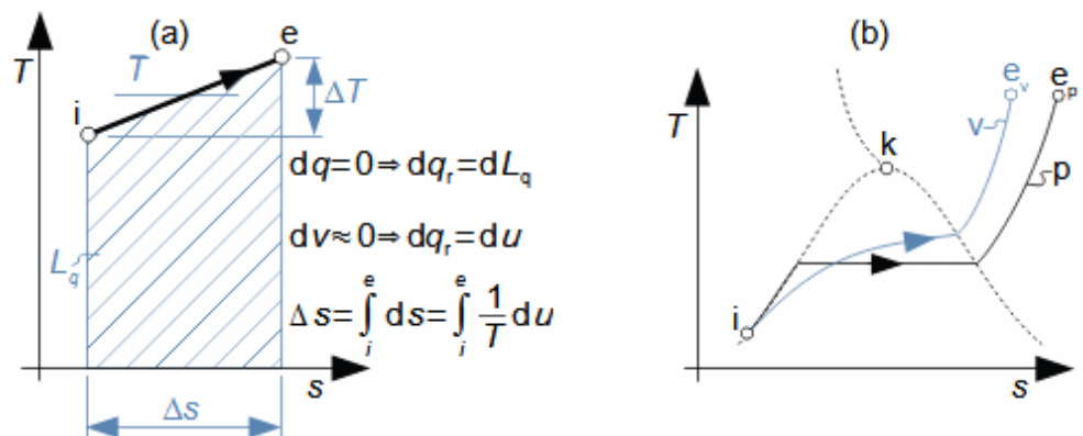
13: Příklady T - s diagramů termodynamických změn
