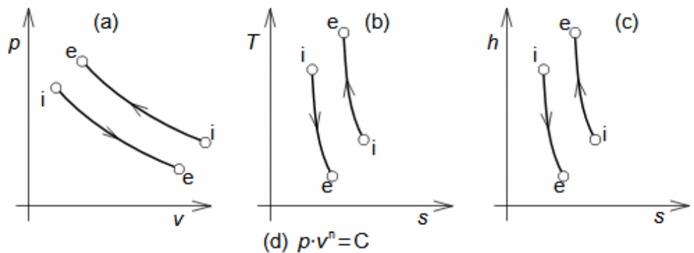
17: Příklady vratných polytropických změn v p - v , T - s a h - s diagramu
