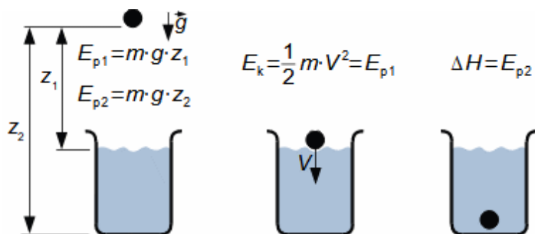
9: Transformace potenciální energie na entalpii
